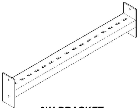
9)U BRACKET
